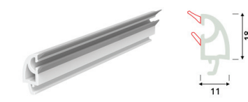
20 MM ÇİFT CAM ÇİTA PROFİLİ
